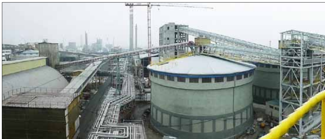
Nová přesýpací věž, dopravníkové a potrubní mosty.
